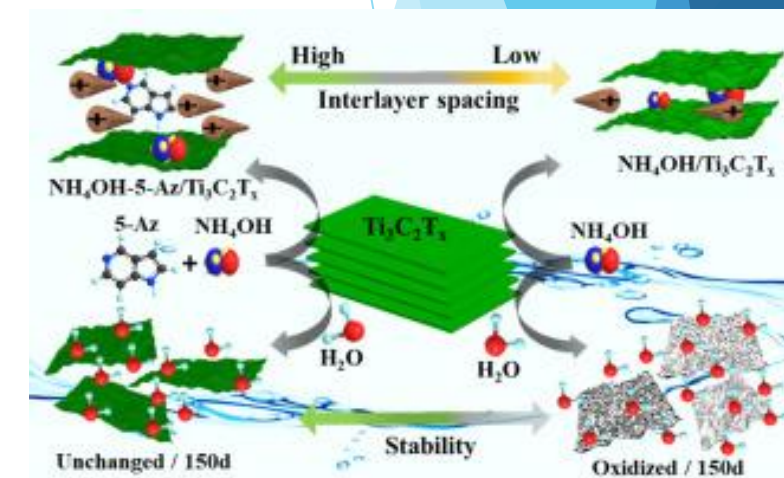
氨輔助雜環胺於 \text{Ti}_3\text{C}_2\text{T}_x MXene 進行軟分層和層間工程，製造穩定的超級電容器
